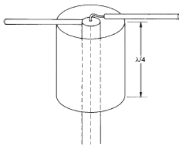
Sleeve Balun 1:1
