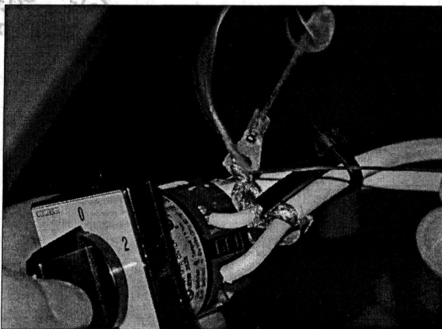
Cinjenje priključkov na stikalo za preklop anten.
