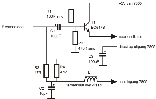
Schema modulator
