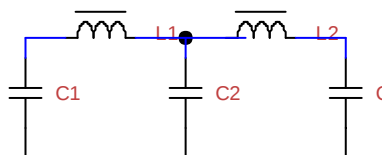
laagdoorlaat filter
