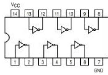
7404
