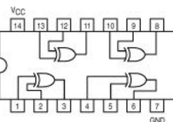
7486
