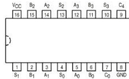
74283
