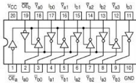
74240
