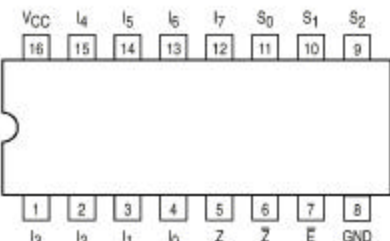
74151
