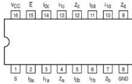
74157
