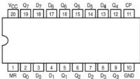
74273
