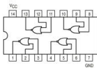
7402
