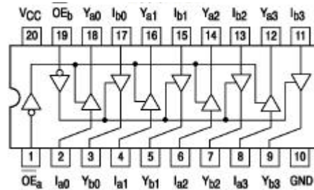
74244
