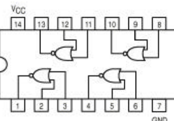
7428
