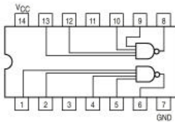
7420
