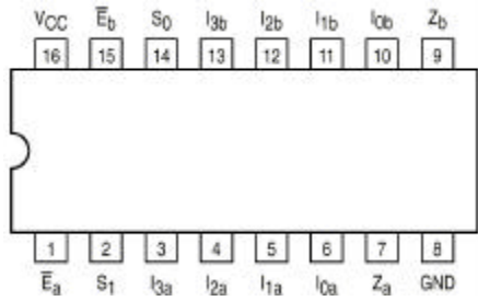
74153
