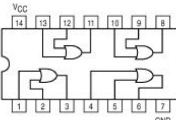
7432
