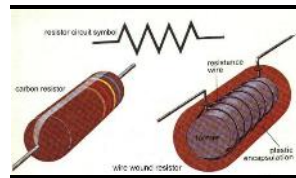
Resistencias, diagrama
