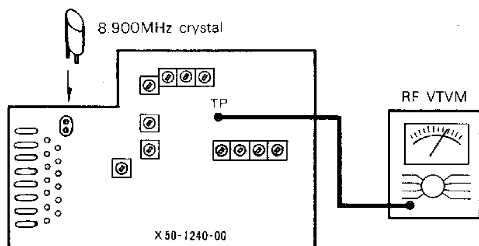
FIG. 6 HET ADJUSTMENT
