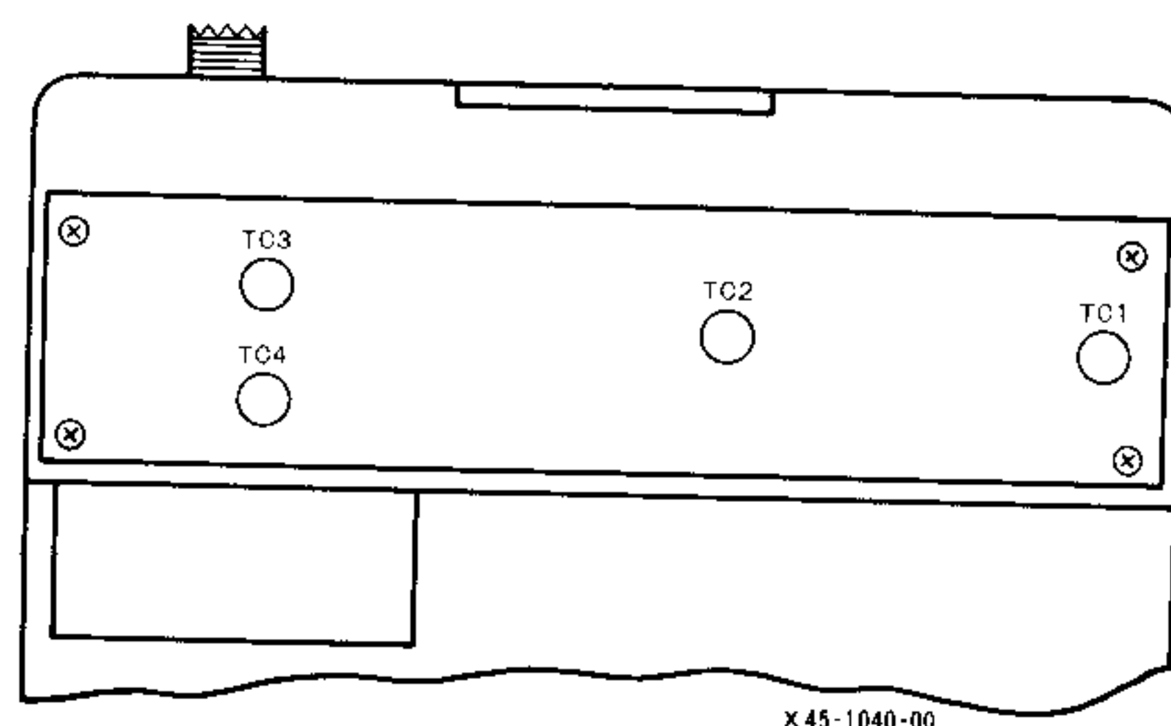
FIG. 10 PA UNIT
