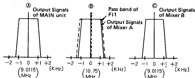
A : P.B. TUNE centered
