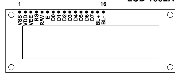
LCD 1602A
