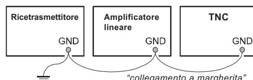
CONNESSIONE DI MASSA IMPROPRIA
