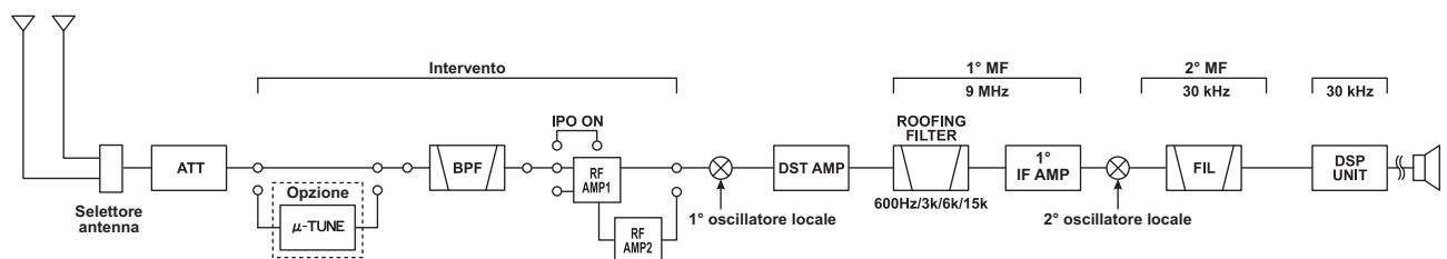
SCHEMA A BLOCCHI STADIO INGRESSO
