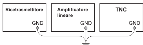
CONNESSIONE DI MASSA CORRETTA
