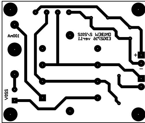
POWSUP Bottom Layer
