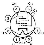
GT-7R(12K7-GT)
