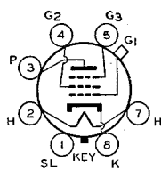
GT-7R (6K7-GT)
