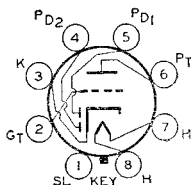
GT-8Q
