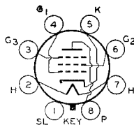
GT-8N
