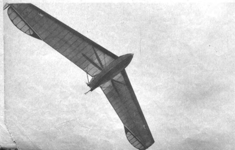
Der „Storch“ hat jetzt am Rumpfe einen 8-PS-Motor erhalten, der ihn vorwärts
