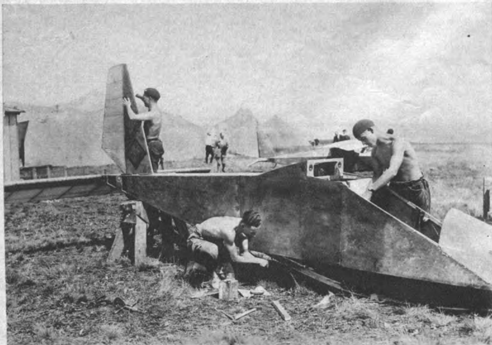
Immer gibt's im Lager etwas zu tun, immer muß geflickt werden. Vor jedem Start wird die Maschine noch einmal gründlich durchgesehen.
