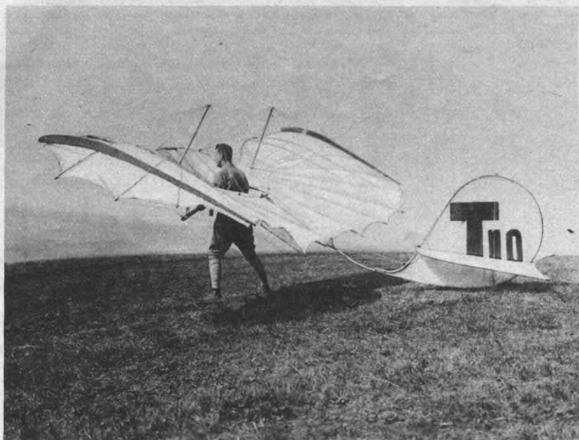
Ein Hängegleiter beim Start. Der Flieger muß selber anlaufen, um auf genügende Geschwindigkeit zu kommen und um im Gleitflug auf den Hang hinunterzuschweben.
