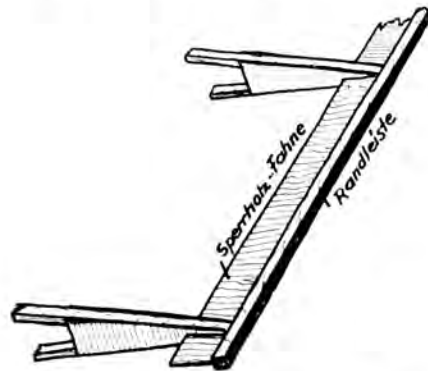
Abb. 65. Randleiste mit Sperrholzfahne.
