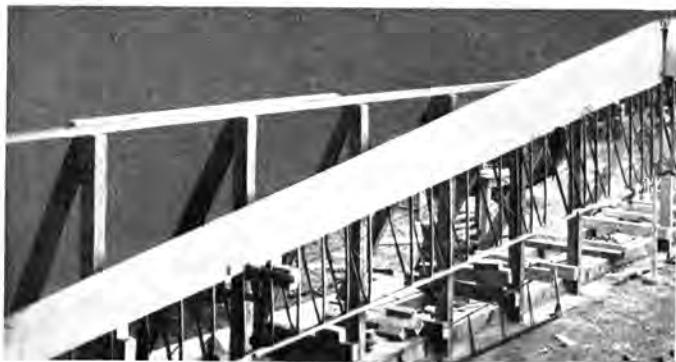
Abb. 38. Helling für senkrechten Flügelbau.
