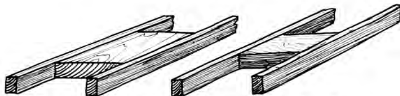
Abb. 57. Füllklöße, wie sie nicht eingebaut werden sollen, da sie keinen weichen Übergang vom Klotz in den Gurt haben.
