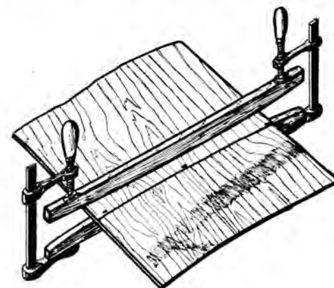
Abb. 12. Preßhölzer zum Verleimen von Schäften.
