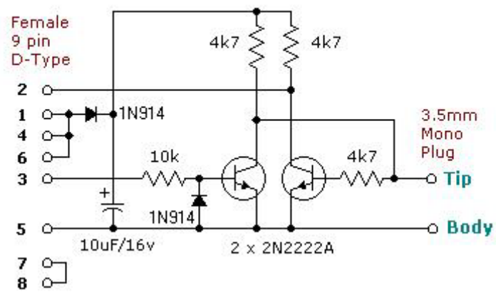
Icom CI-V Interface
