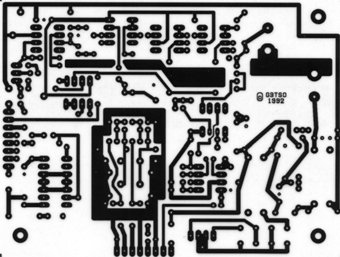
G3TSO EXCITER MODULE 1 - SL1621
