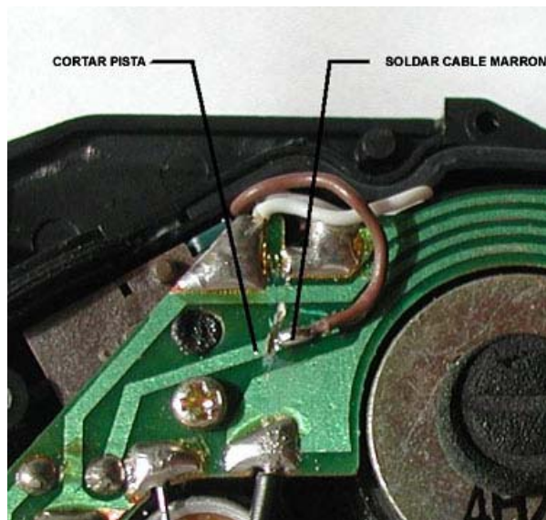
Modificación de la placa de circuito impreso
