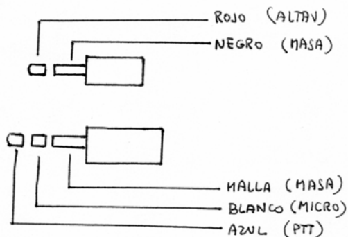
CONEXIONES JACKS
