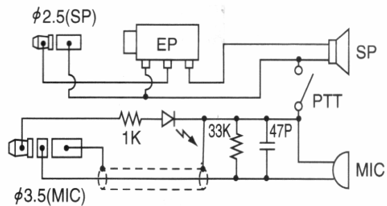
ESQUEMA ORIGINAL MICRO
